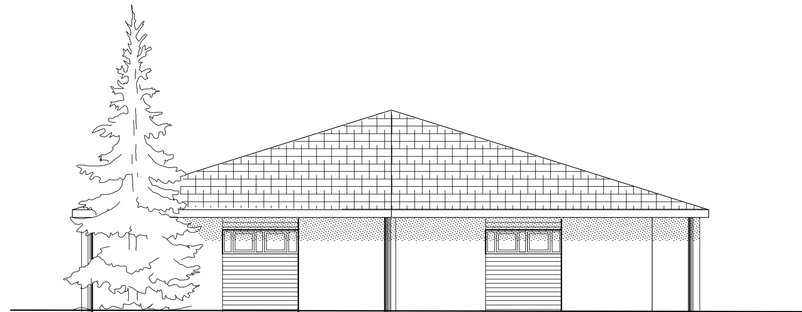
Ansicht West
